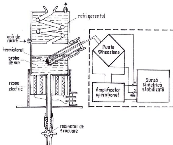
Fig. 4. Ebulliometru – schemă de principii (CAV)
